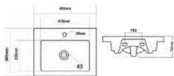
Avante Mini Dimensions : 450x360x120mm G3715PW Basin
